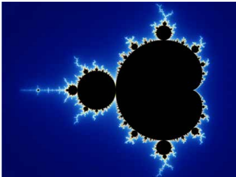
Conjunto de Mandelbrot (Imagen: Wolfgang Beyer usando el programa Ultra Fractal 3)
